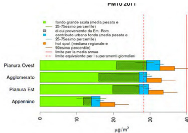
Figura 5.3.3 - Ripartizione dell'origine dell'inquinamento per aree geografiche da PM10 (linea rossa tratteggiata = VLE di 28 µg/m3 e linea rossa continua VL annuale = 40 µg/m3)
