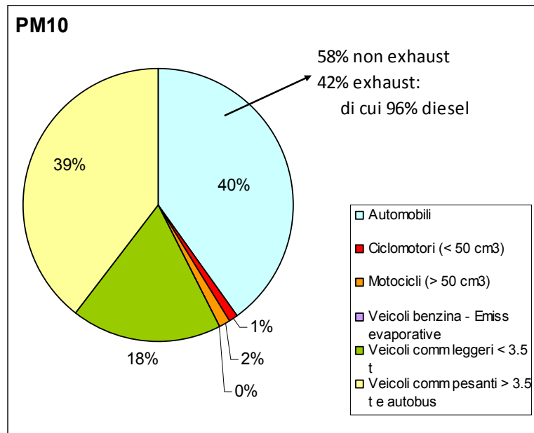
Figura 9.2.2 - Ripartizione dei contributi emissivi di PM10 per tipo di veicolo in Regione (exhaust: emissioni derivanti dalla combustione, non-exhaust = emissioni derivanti dall'usura freni, pneumatici e abrasione strade)
